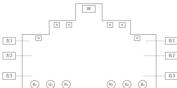
図 1 ステージ照明配置図
